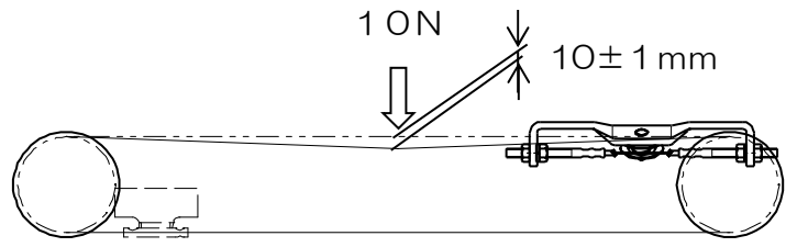
高速戸と低速戸を連動するワイヤロープのたわみ量測定位置
